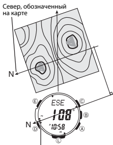
Указание севера цифровым компасом
